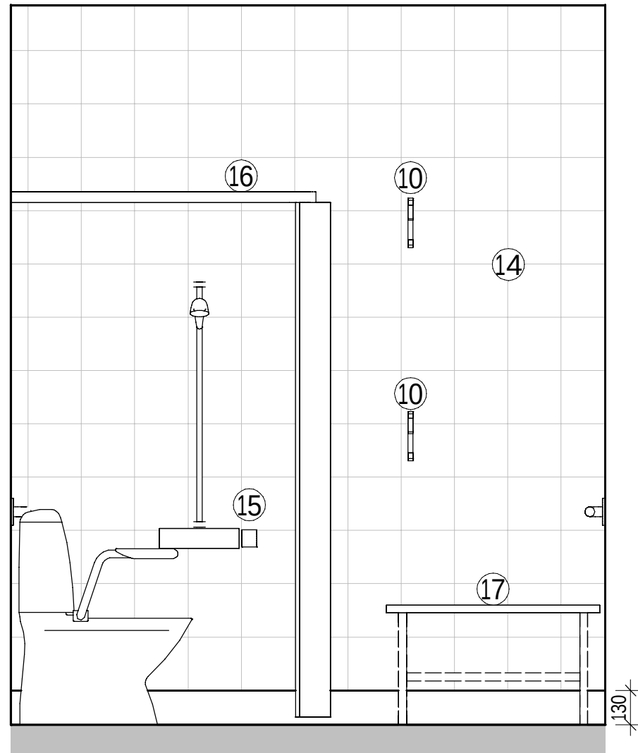
ELEVATION RWC/D 1016-B 1 : 20
