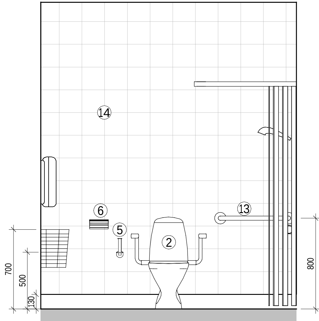
ELEVATION RWC/D 1016-A 1 : 20
