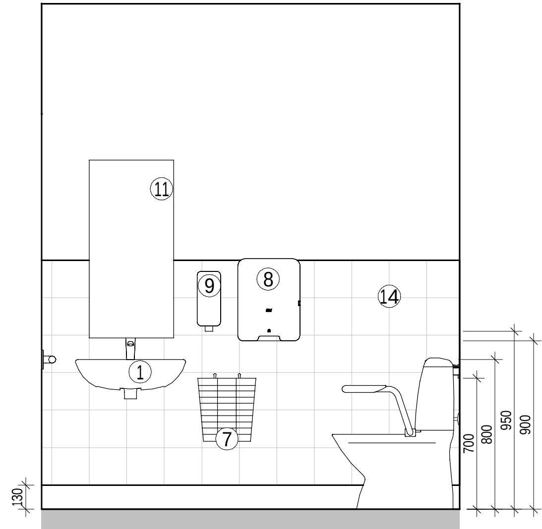
ELEVATION RWC/D 1016-D 1 : 20
