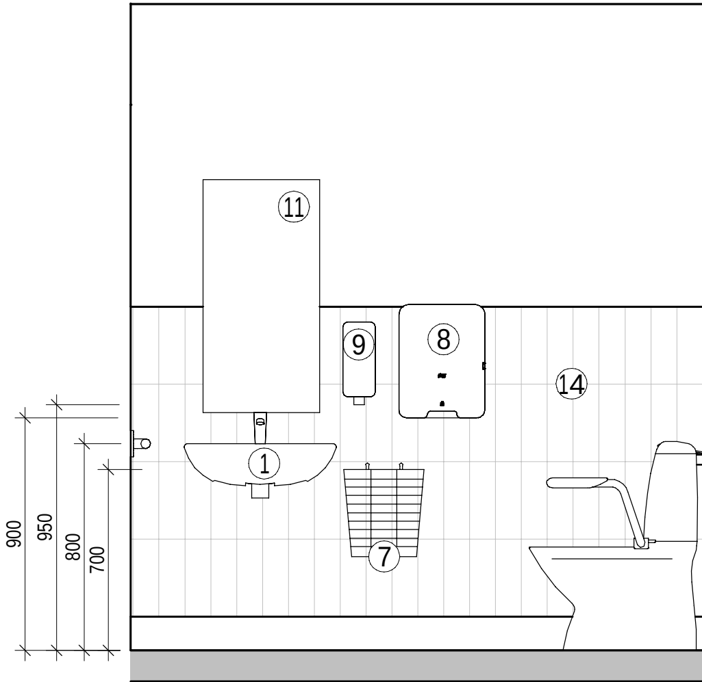
ELEVATION RWC 1007-D 1 : 20
