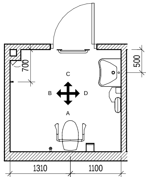
PLAN RWC 1007 1 : 50
