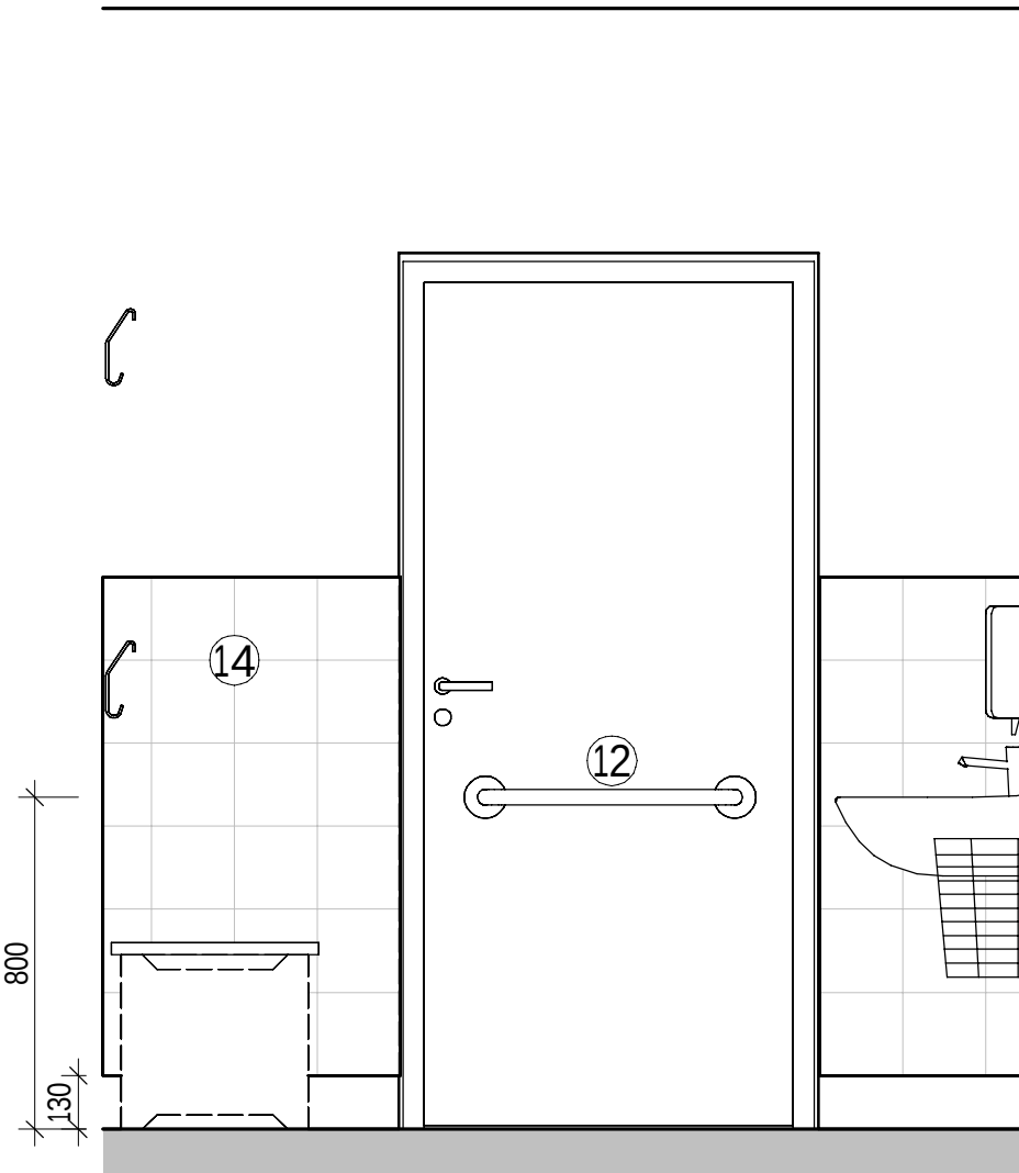
ELEVATION RWC/D 1016-C 1 : 20
