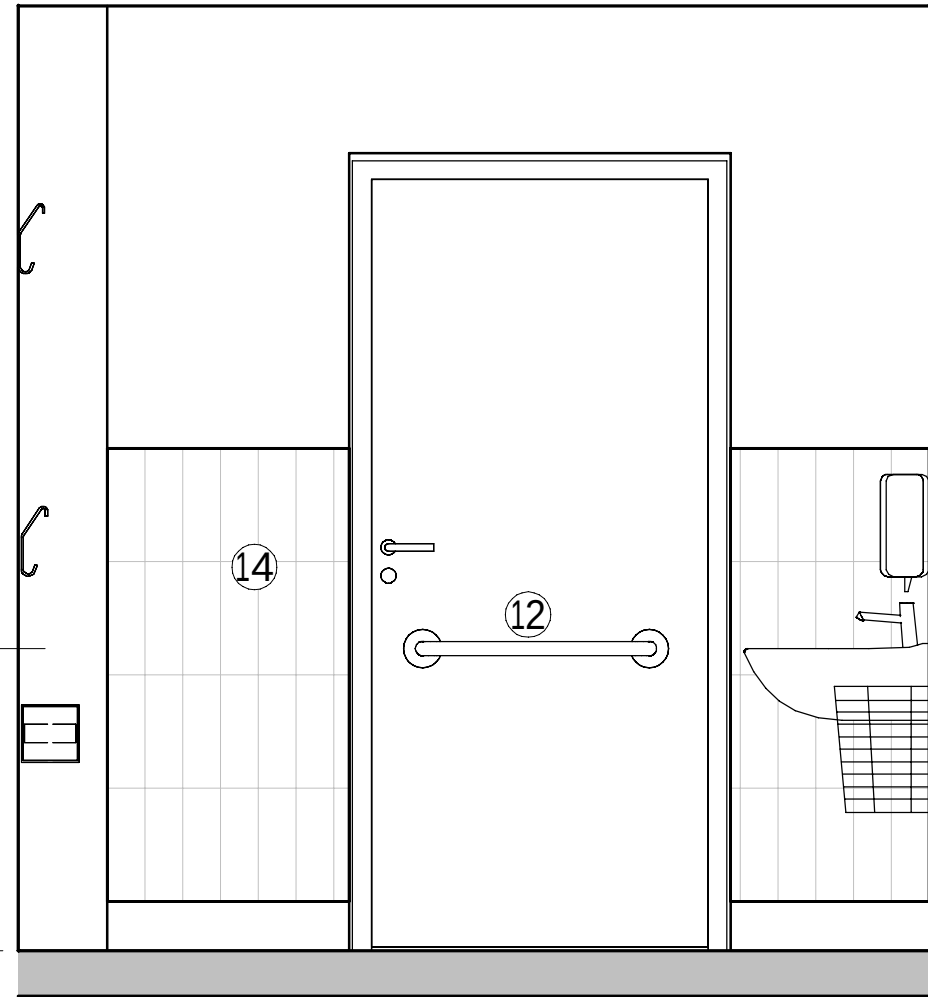
ELEVATION RWC 1007-C 1 : 20
