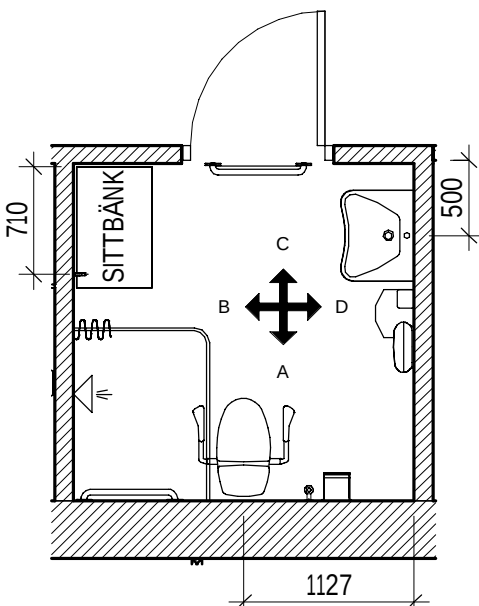
PLAN RWC/D 1016 1 : 50
