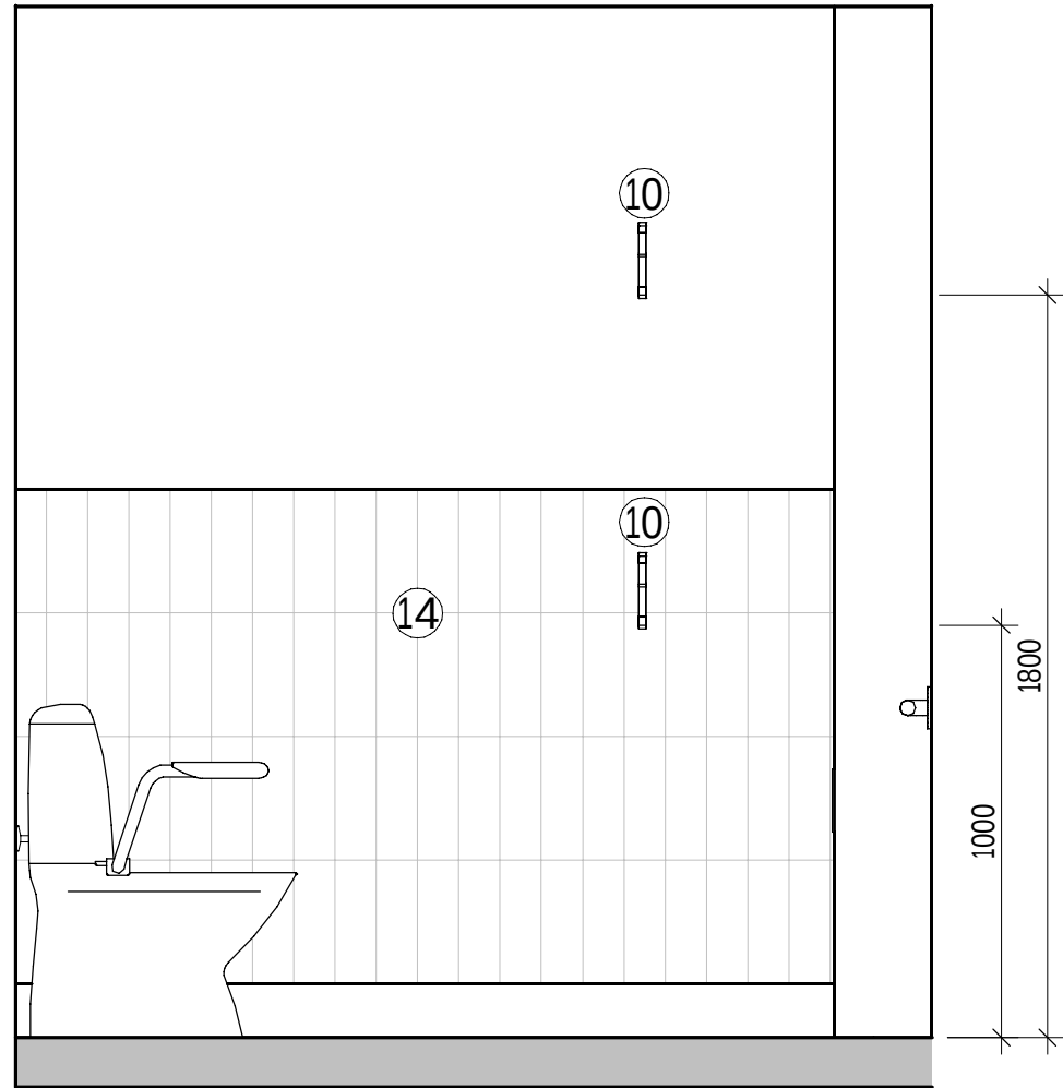
ELEVATION RWC 1007-B 1 : 20
