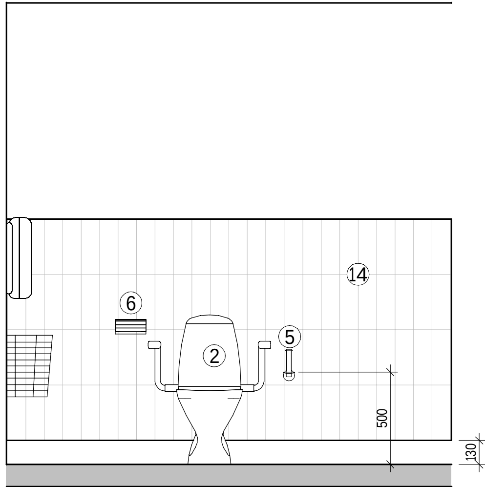
ELEVATION RWC 1007-A 1 : 20
